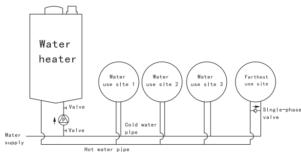
Fig.2 Usage Scenario 1
